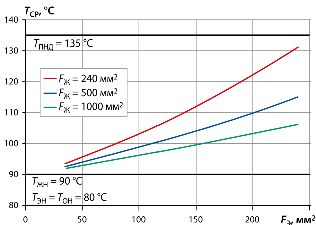
Средняя температура кабеля после его прогрева теплом от жилы и экрана (конец 3-го этапа)
