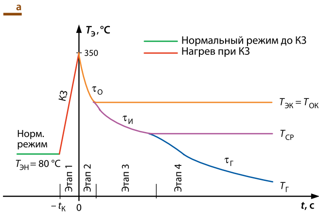
• Рис. 1. Температура экрана (а) и оболочки (б) до короткого замыкания и после него
