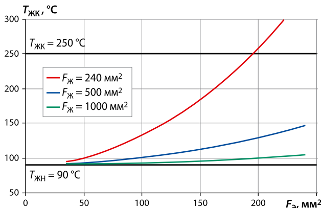
• Рис. 2. Температура жилы в момент отключения короткого замыкания (конец 1-го этапа)
